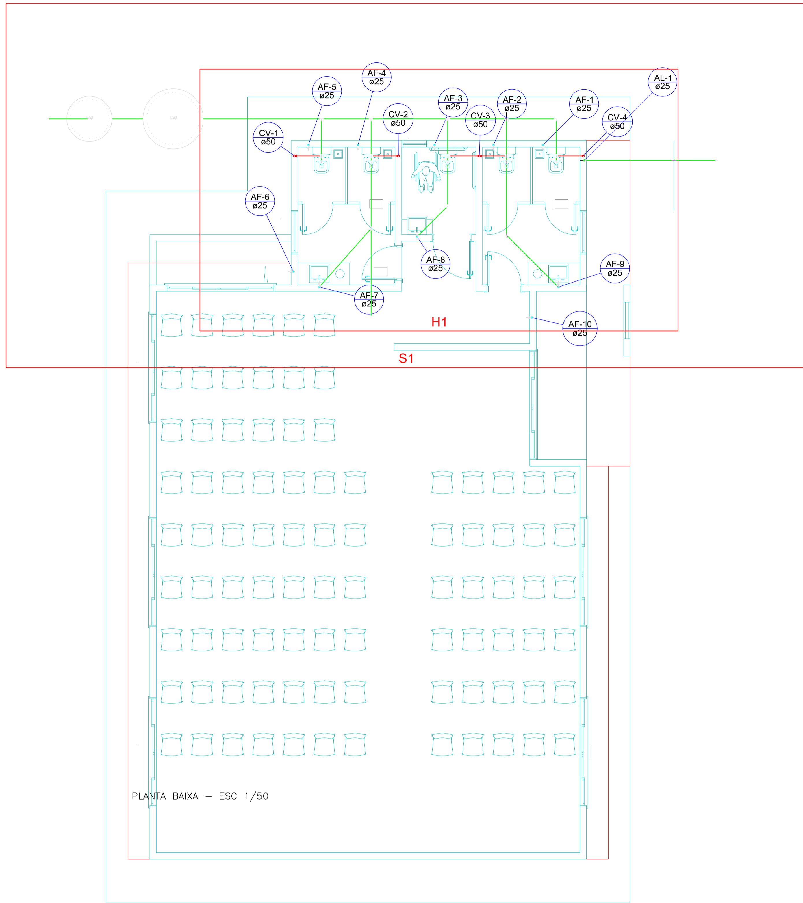
PLANTA BAIXA TÉRREO – ESC 1/50
