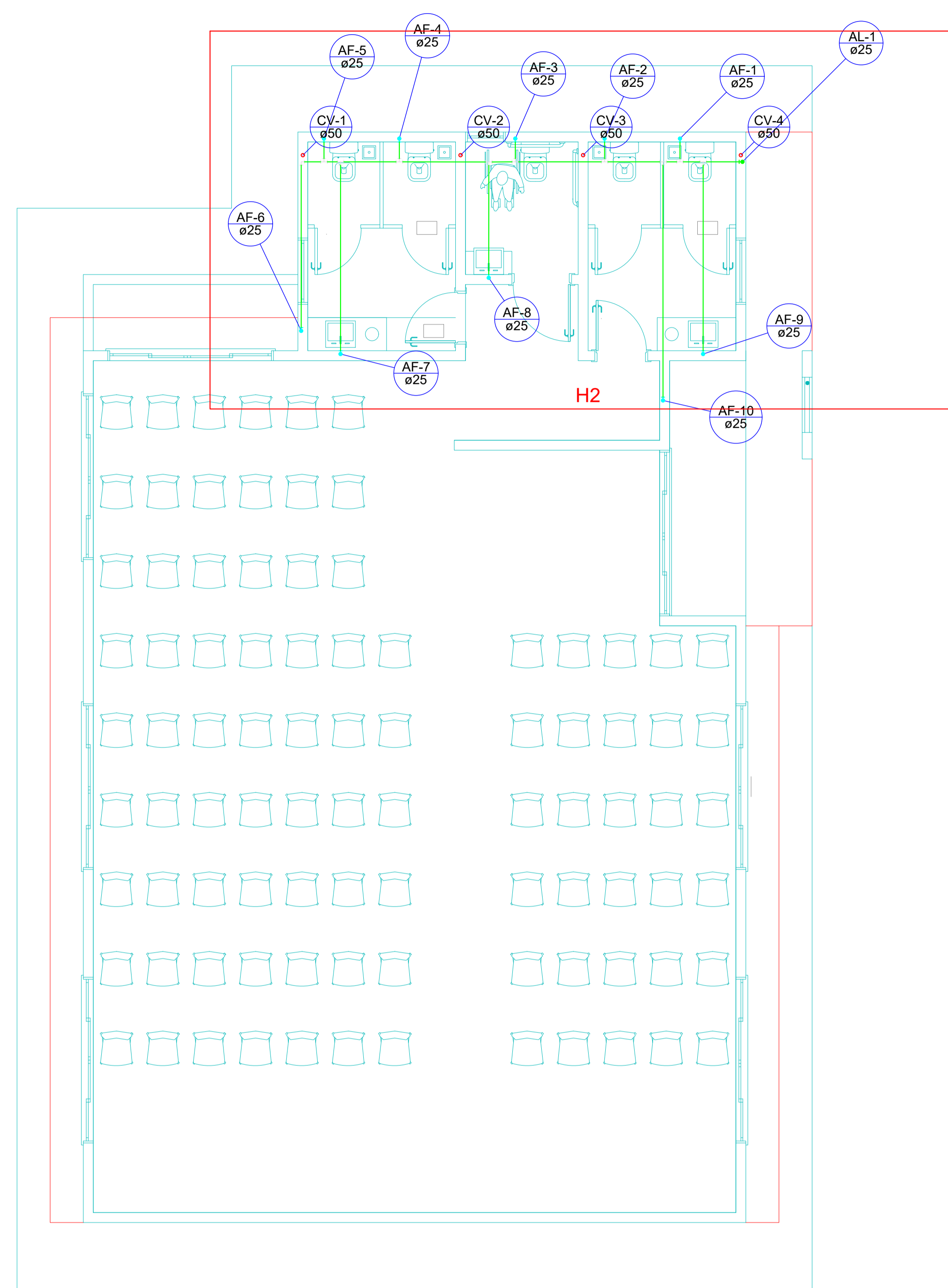
PLANTA BAIXA BARRILETES – ESC 1/50
