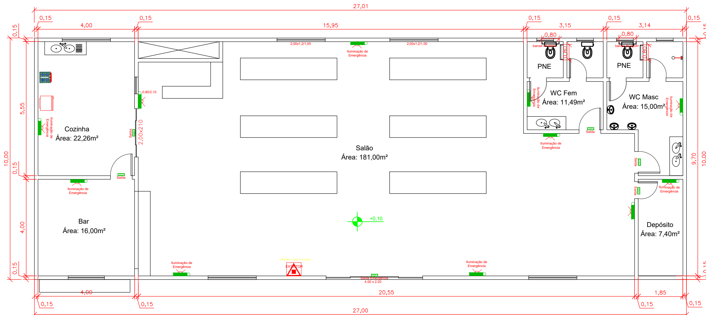
Planta Baixa Escala: 1/100
