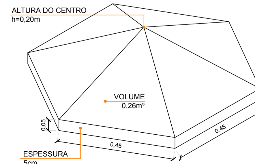
T1 DETALHE CHAPÉU CHINÊS ESC. 1/10
