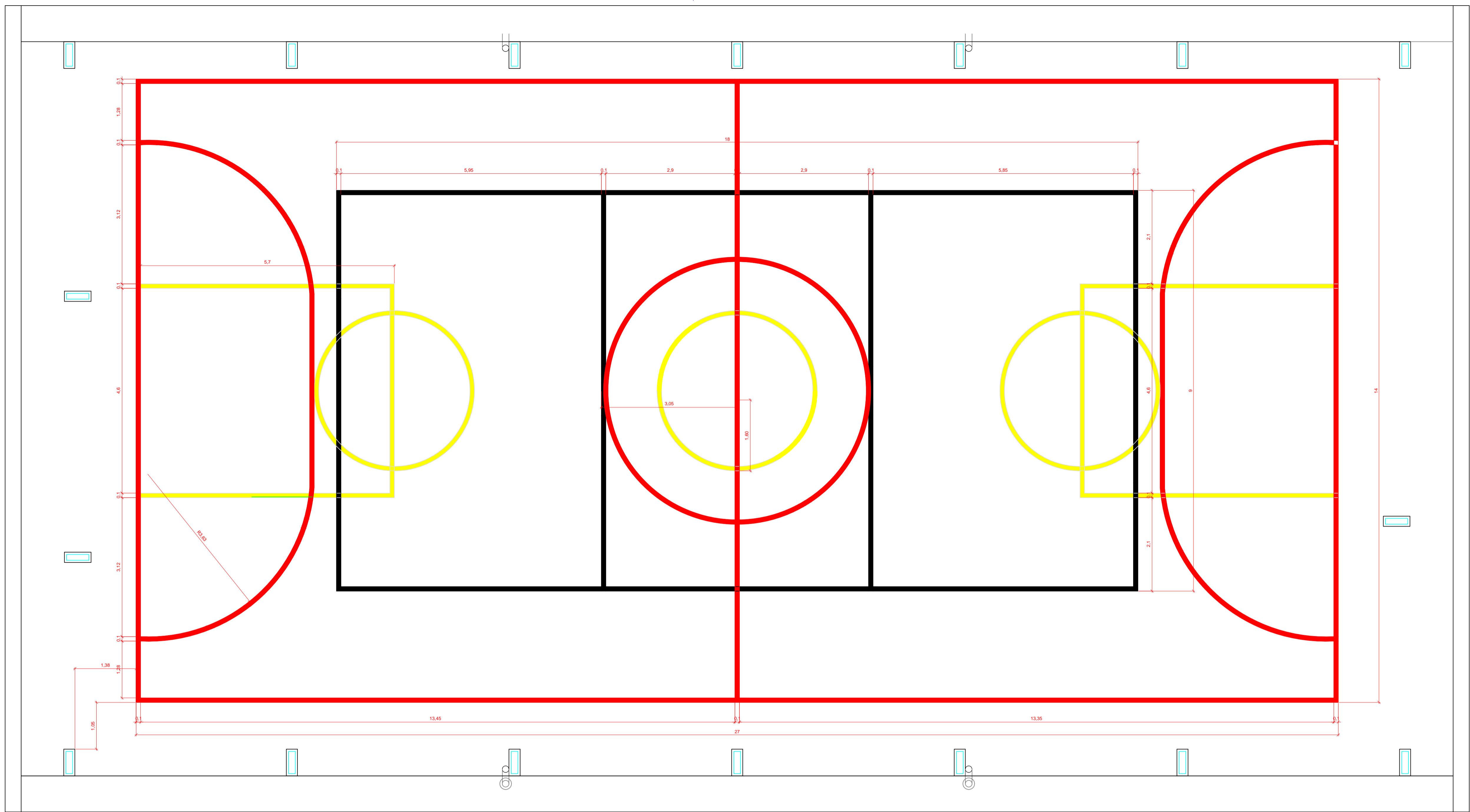
PLANTA DE DEMARCAÇÃO DA QUADRA - ESC 1/50
