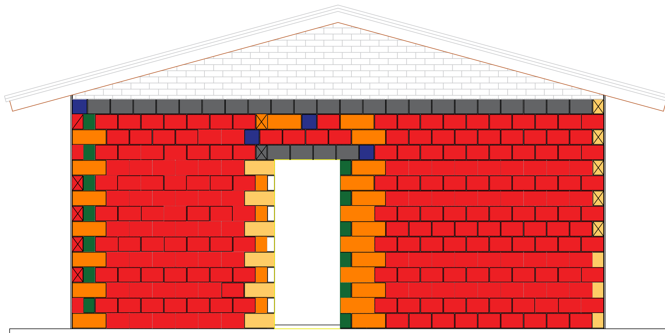
PLANTA PAGINAÇÃO VISTA 02 ESCALA 1:30
