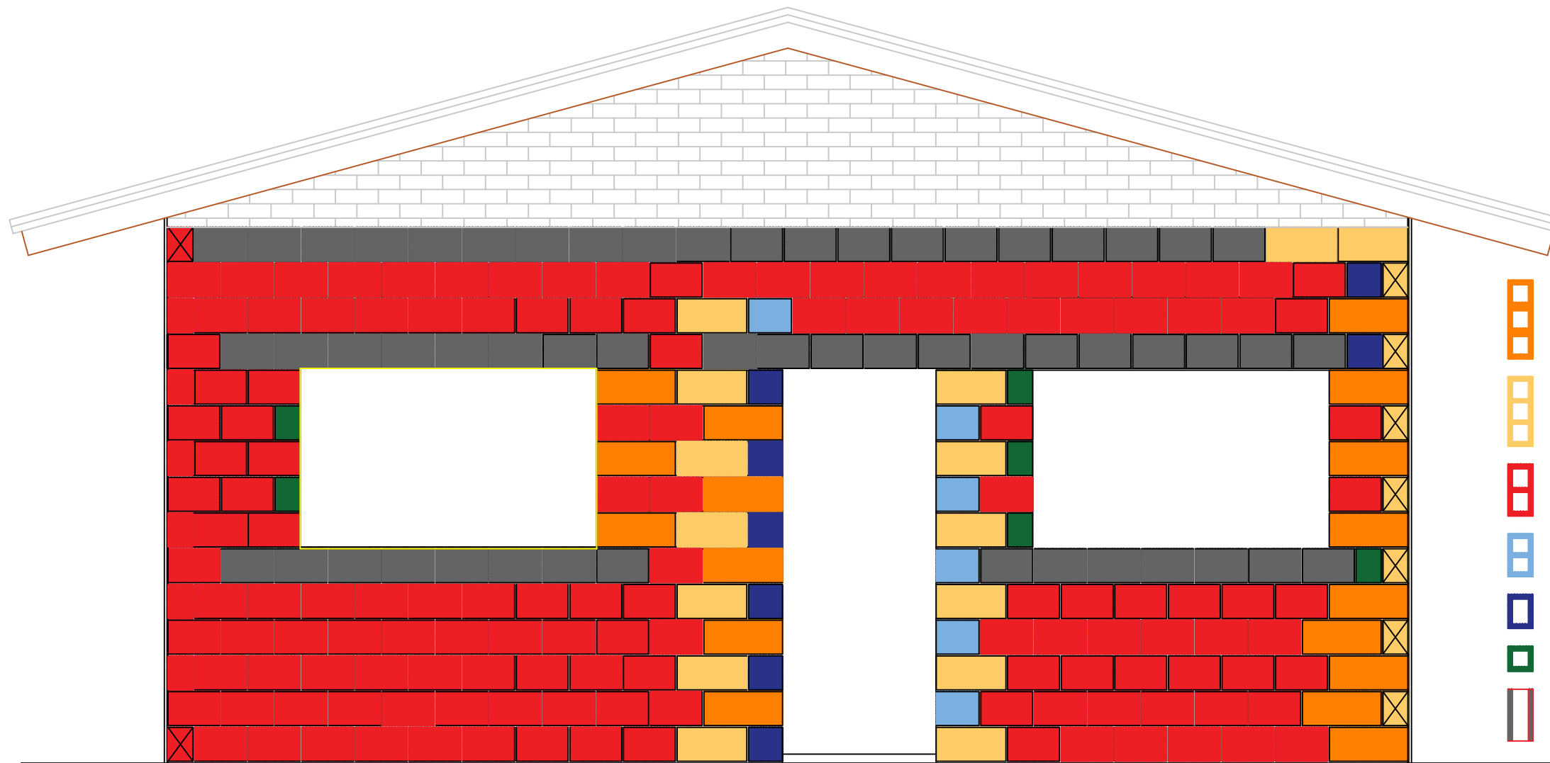
PLANTA PAGINAÇÃO VISTA 01 ESCALA 1:30
