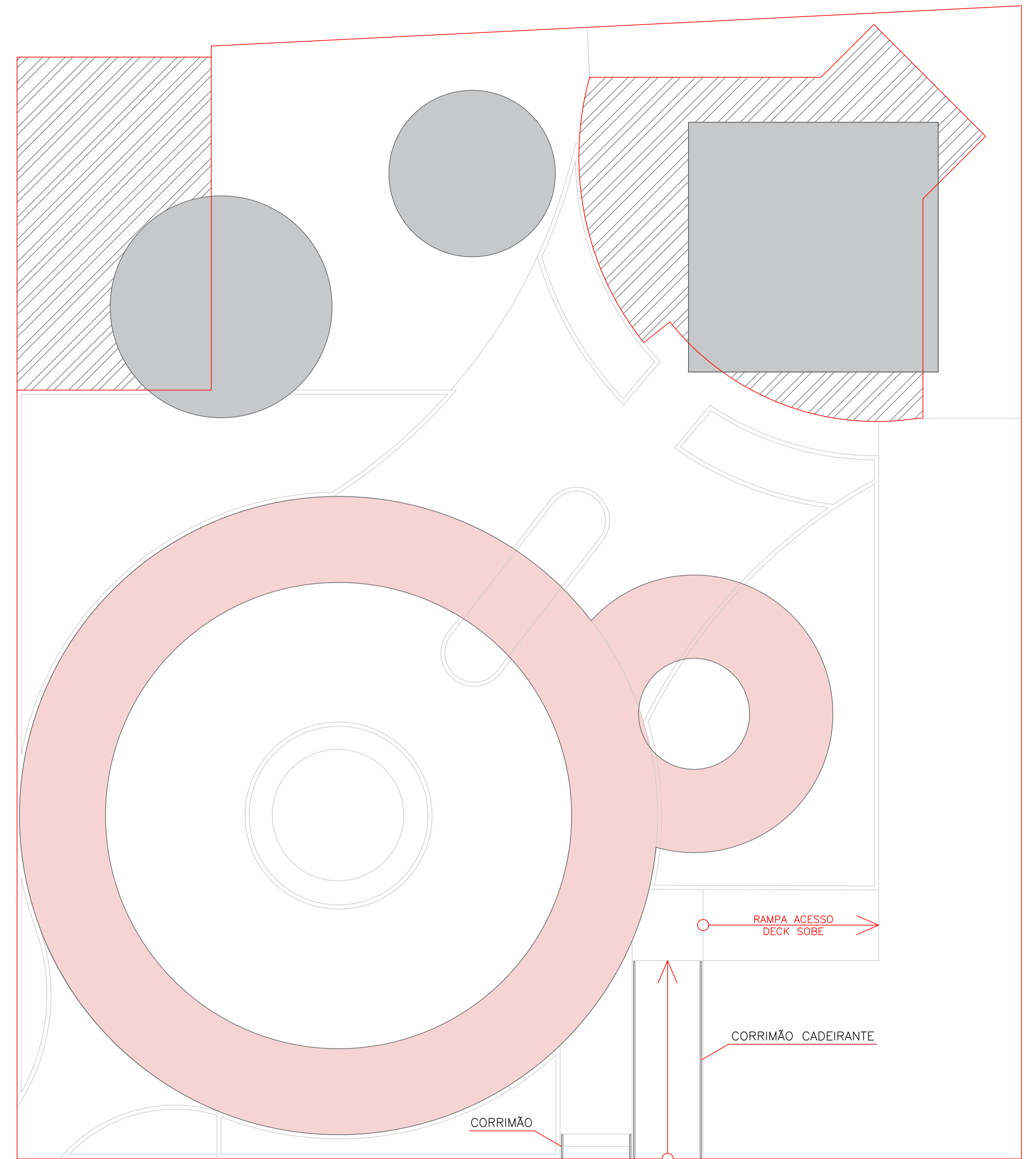
PLANTA DEMOLIR/ REMOVER/ CONSTRUIR TERRENO MUNICIPAL ESCALA 1:100
