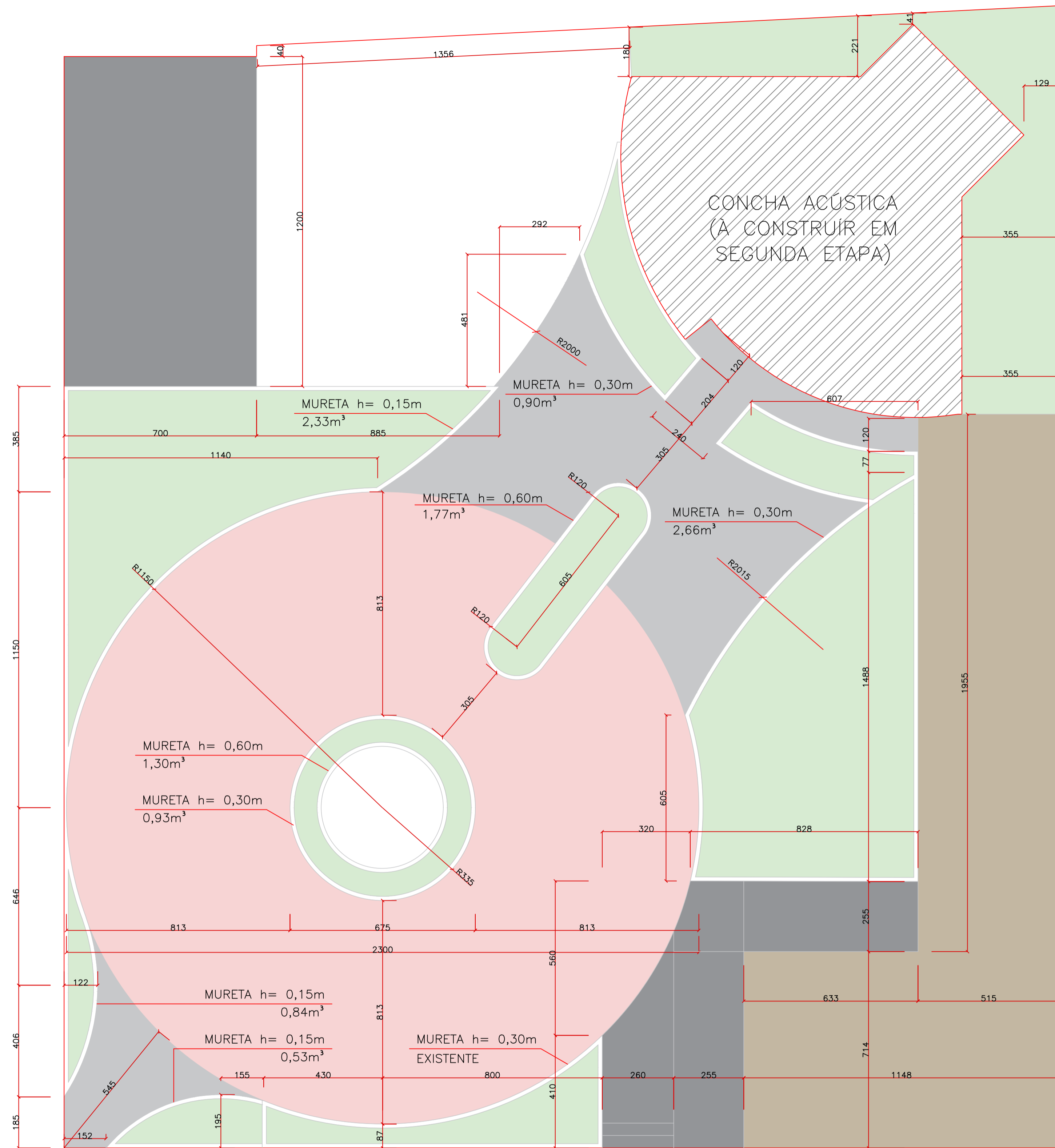
PLANTA DE PAGINAÇÃO DE PISOS E DIMENSIONAMENTOS TERRENO MUNICIPAL ESCALA 1:100
