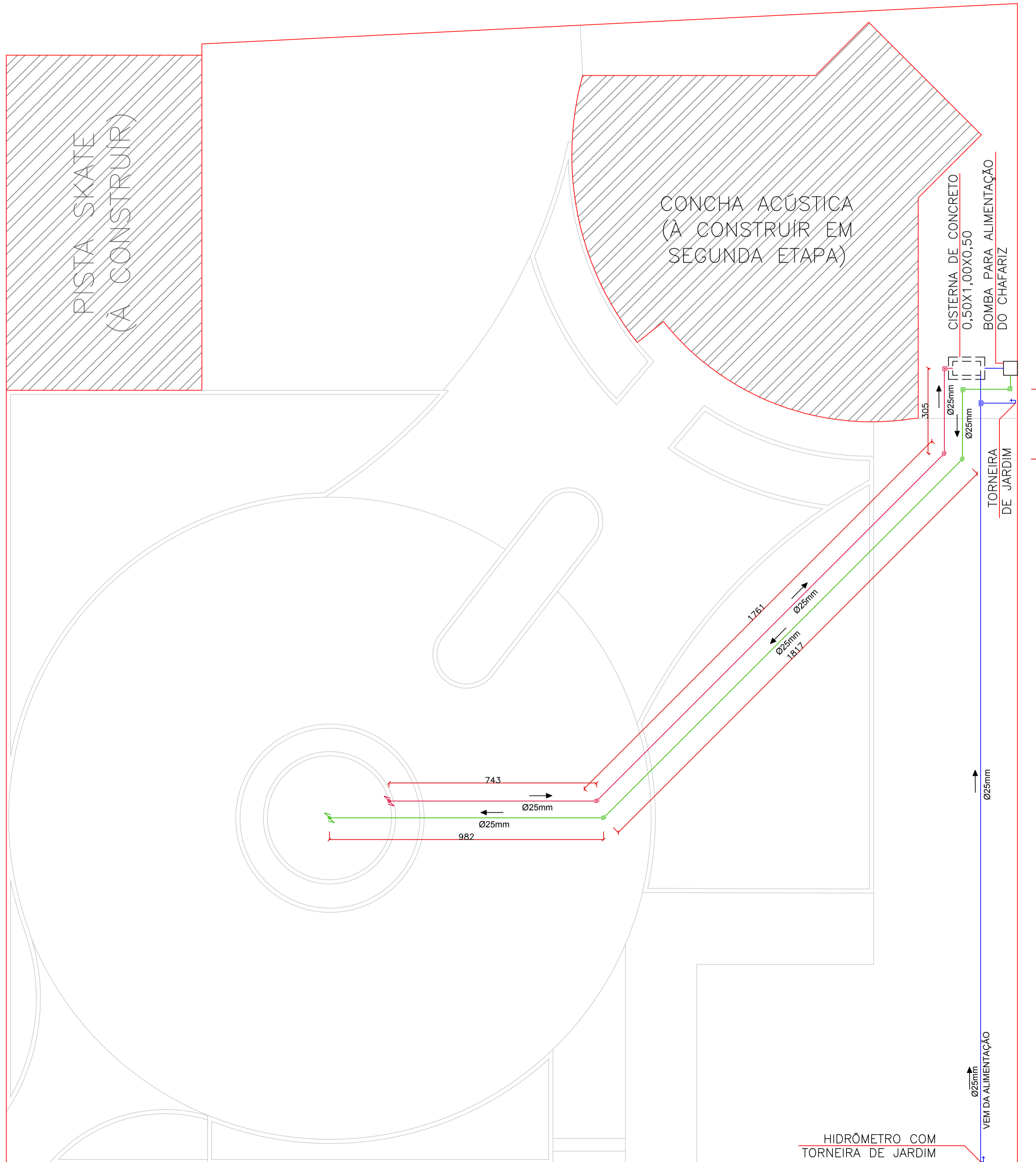
PLANTA HIDRÁULICA DO CHAFARIZ TERRENO MUNICIPAL ESCALA 1:100
