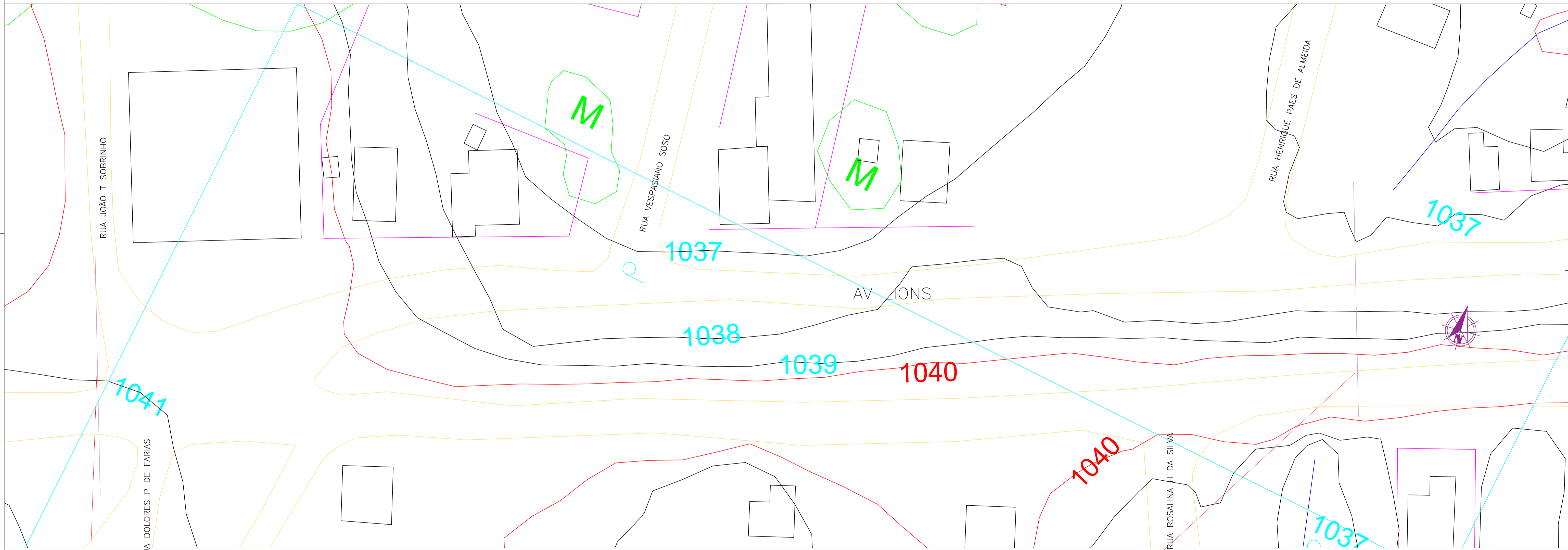
PLANTA PLANIALTIMÉTRICA – ESC 1/300
