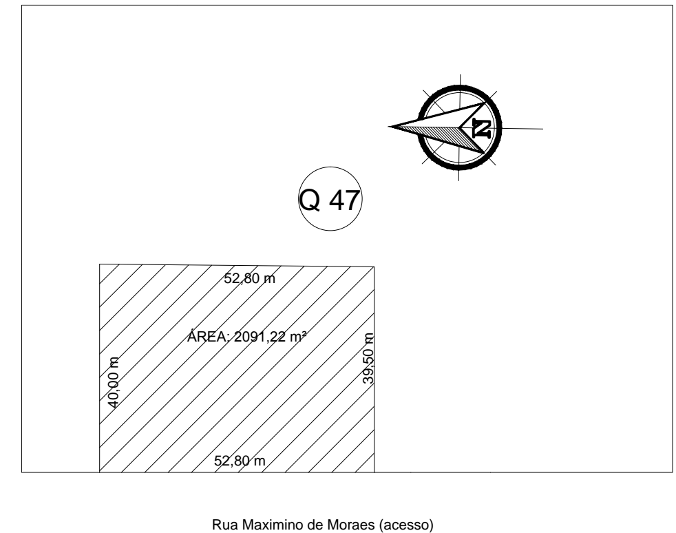
PLANTA DE SITUAÇÃO - 1/1000
