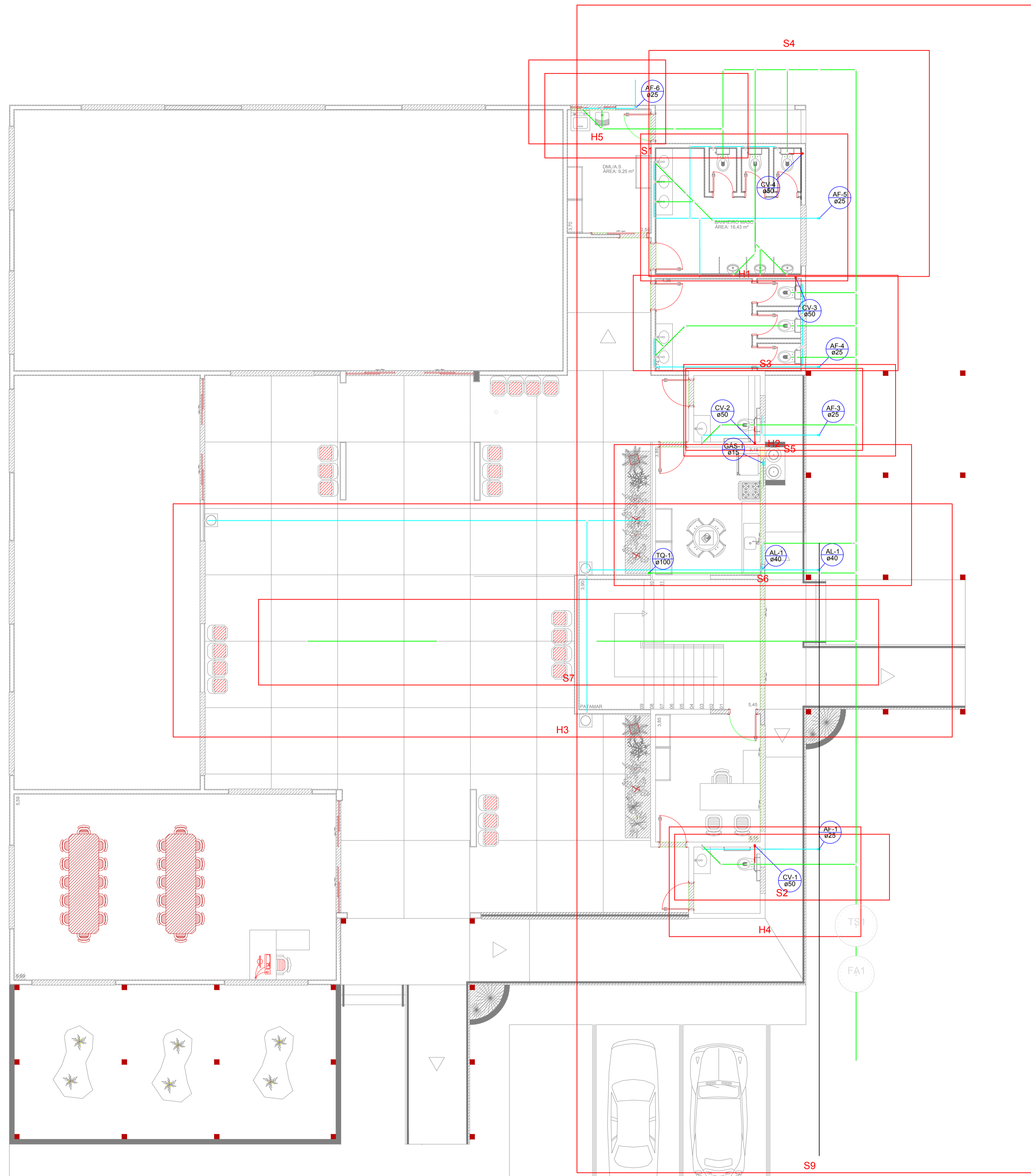
PLANTA BAIXA TERREO - ESC 1:75
