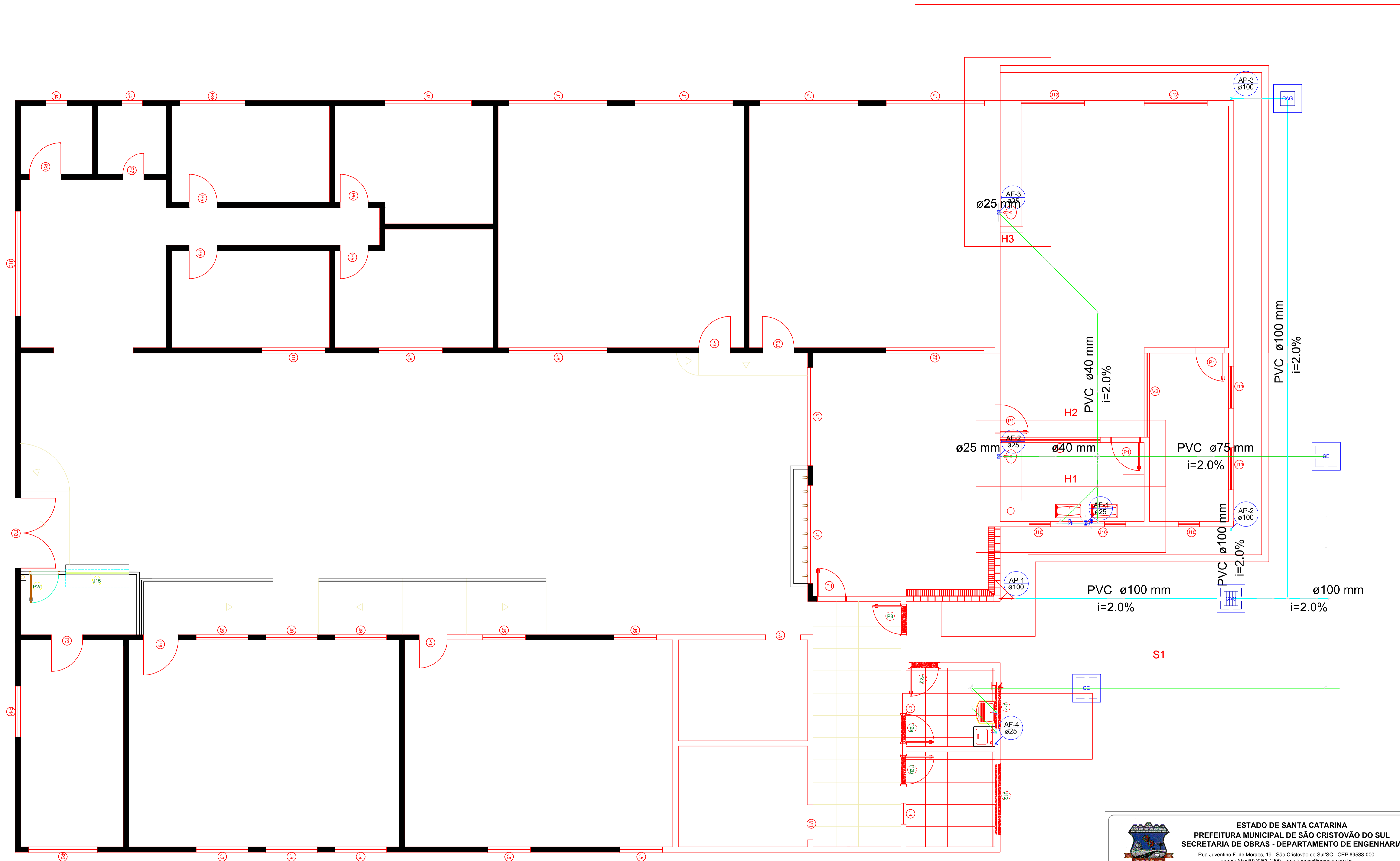
PLANTA BAIXA ESC: 1/50
