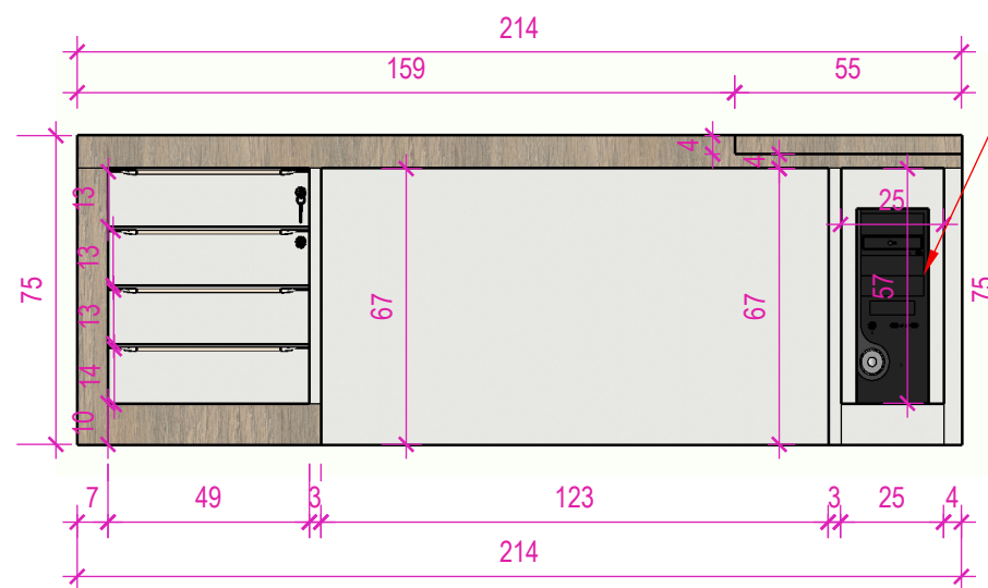
MESA INTERNA ESC: 1/20
