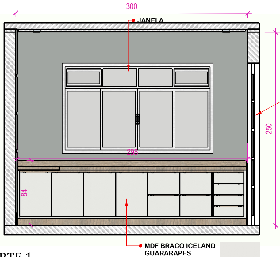
CORTE 1 ESC: 1/30
