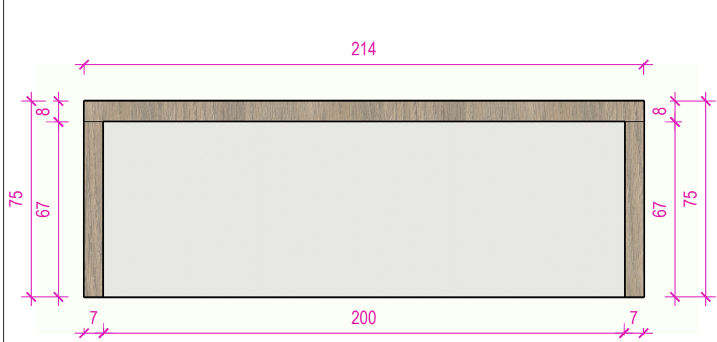
MESA FRONTAL ESC: 1/20
