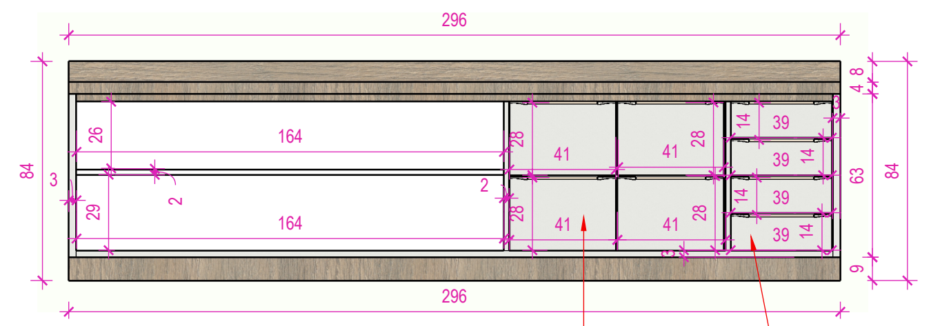
BALCÃO-INTERNO ESC: 1/20
