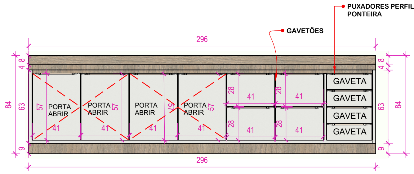
BALCÃO ESC: 1/20
