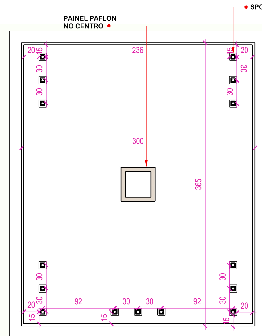
PLANTA ILUMINAÇÃO ESC: 1/30
